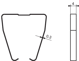
18FF-H1 (metallic retainer)
